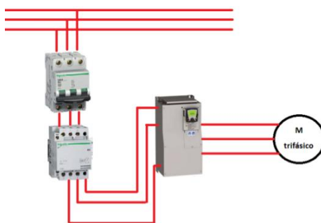
Figura 7. Diagrama de solução industrial. Fonte: do autor (2012).
