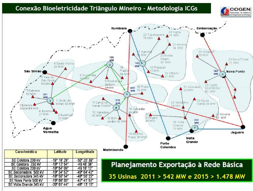
Figura 8: Conexão Bioeletricidade no Triângulo Mineiro. Fonte: COGEN (2010)
